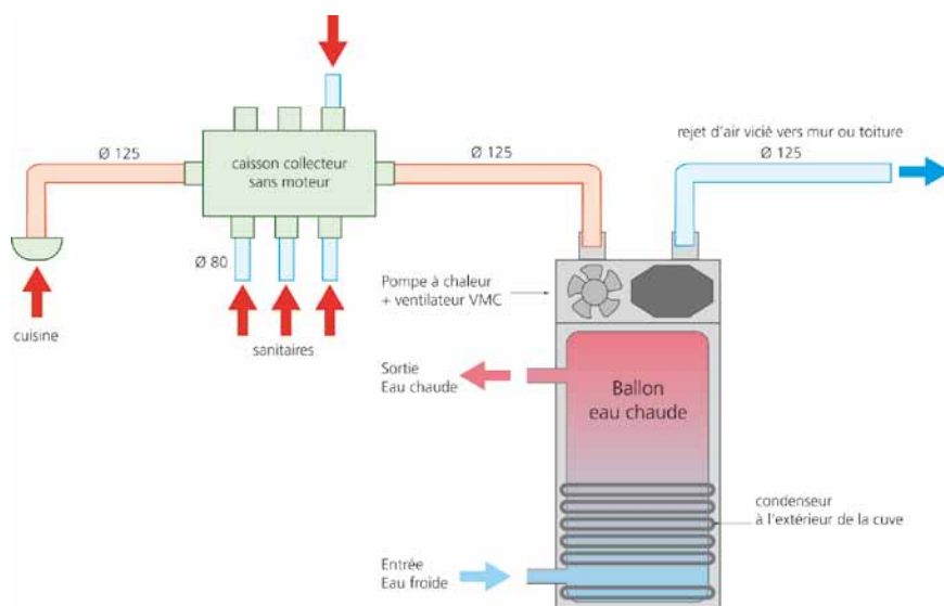
Shéma d'installation (dimension en mm)
